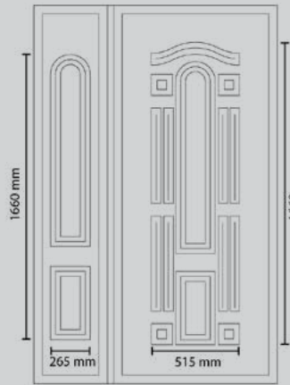
Maße mit Toleranz
