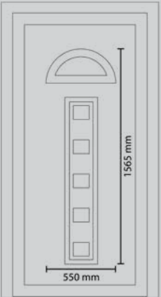
Maße mit Toleranz
