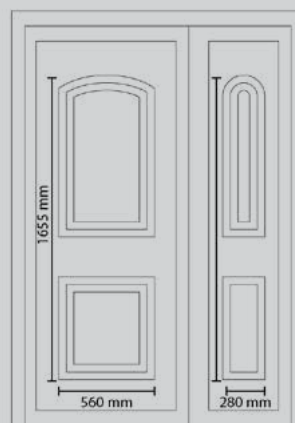
Maße mit Toleranz
